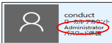
＜Windows8.1、Windows10 の例＞
