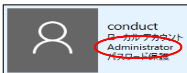
<Windows8.1、Windows10 の例>
